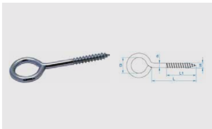
Ringschraube Art. 001 galv. Verzinkt
