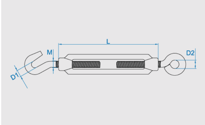
Spannschloß Art. 077 Edelstahl
