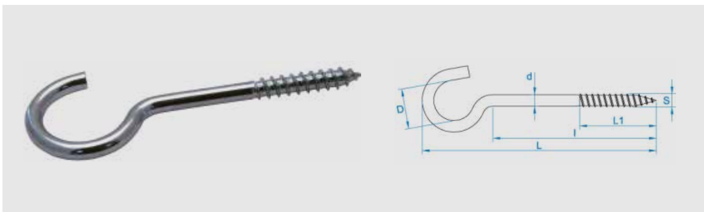
Gebogene Ringschrauben Art. 011 galv. Verzinkt
