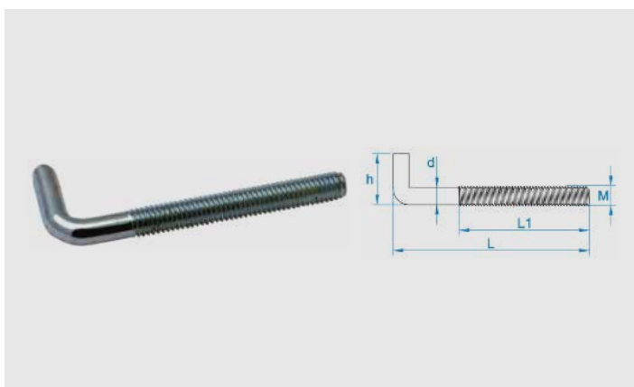
Schraubhaken Art. 027 galv. Verzinkt
