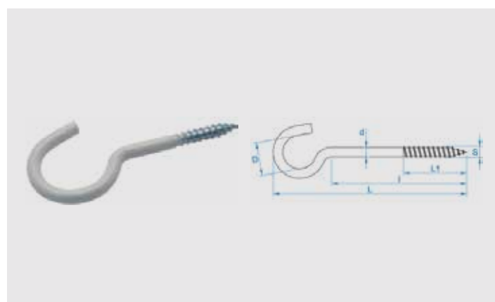
Gebogene Schraubhaken Stahl, Pulverbeschichtet weiß
