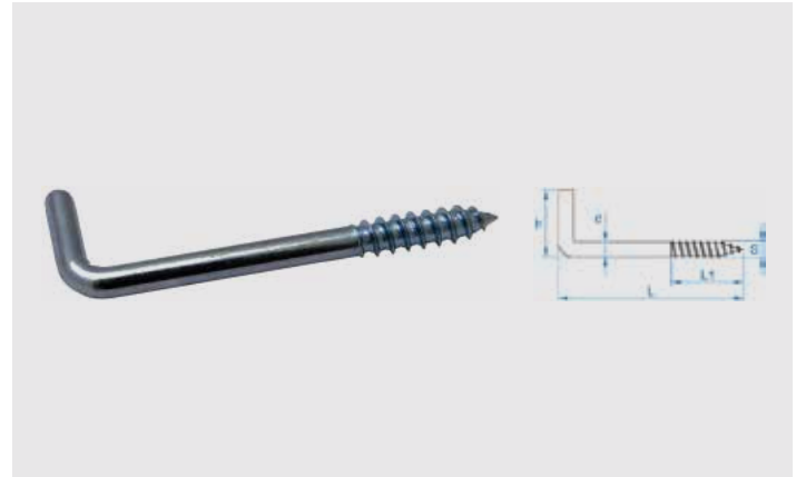
Gerade Schraubhaken Art. 007 galv. Verzinkt
