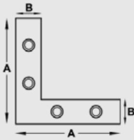
Flachwinkel Stahl verzinkt
