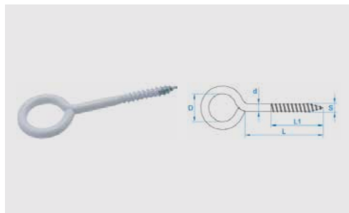
Art. 001 Stahl, Pulverbeschichtet weiß
