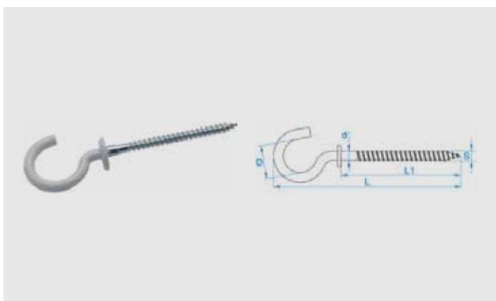
Gebogene Schraubh. mit Befle Art. 014 Stahl, pulverbeschichtet weiß
