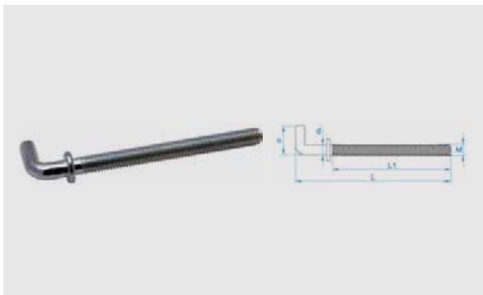
Schraubhaken Art. 019 galv. Verzinkt
