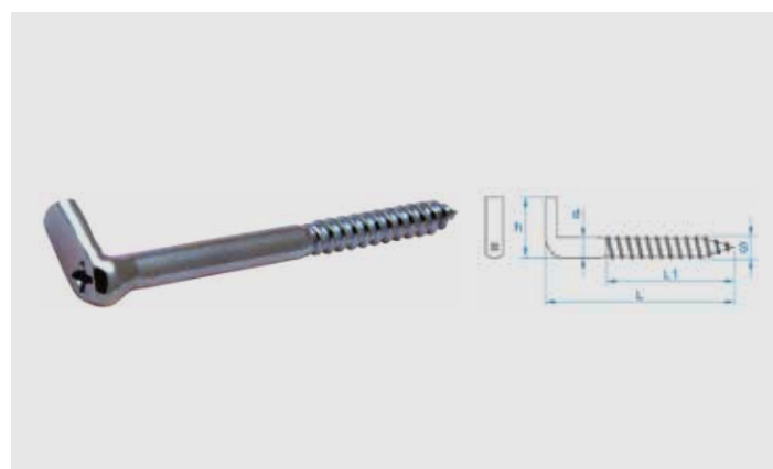
Kreuzschlitzhaken Art. 009 galv. Verzinkt PH2
